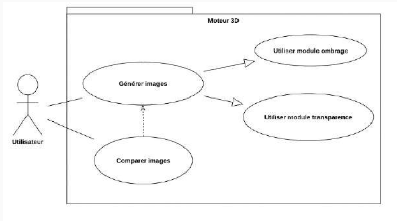
Figure 2: Cas d'utilisation
